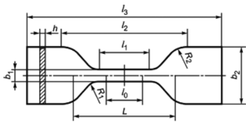
Рисунок ДБ.1 - Образец для испытания
