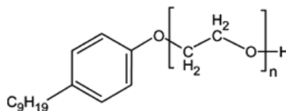
Рисунок ДА.1 - Формула детергентов нонилфенолаэтоксилата (CAS N 9016-45-9)
